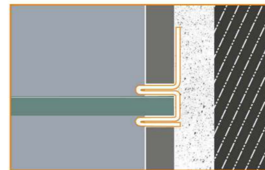
Instalación Vertical en Pared Vertical Installation on Wall
